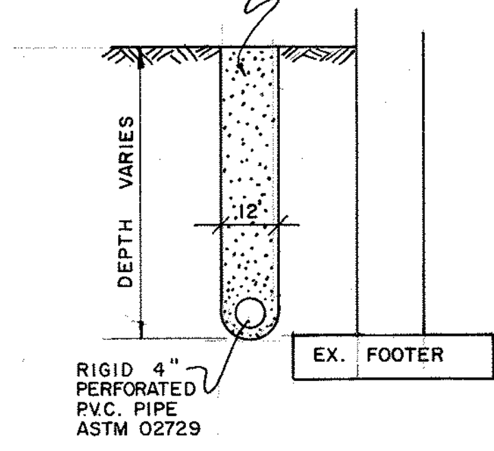
FOOTER DRAIN DETAIL (N.T.S.)
