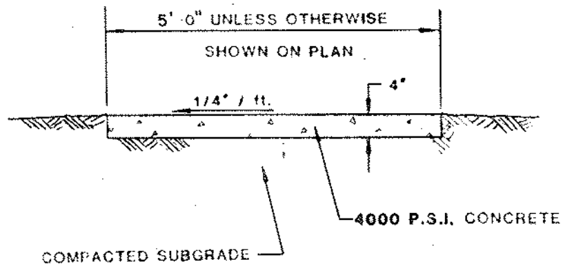
TYPICAL SIDEWALK DETAIL (N.T.S.)
